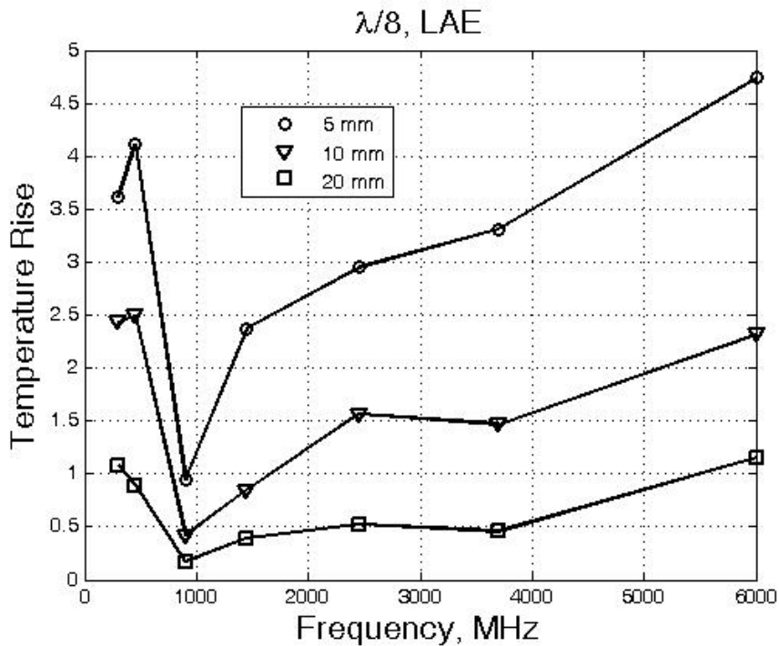
სურ. 4.3.2 ტემპერატურის დამოკიდებულება სისშირეზე.
