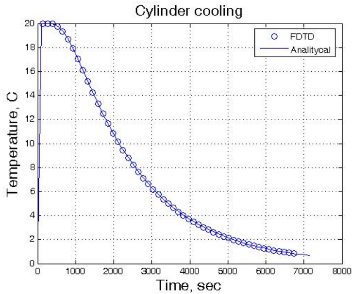
სურ 3.7.1 რიცხვითი ამონახსნის შედარება ანალიზურთან.
