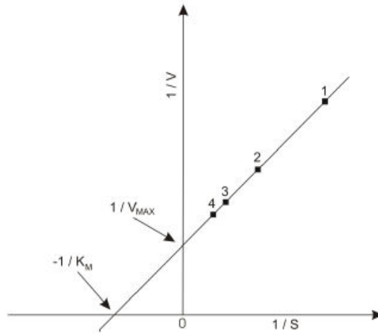
სურათი 2.4. შებრუნებულ ლაინუივერ-ბერკის კოორდინატებში აგებული რეაქციის სიჩქარის დამოკიდებულება სუბსტრატის კონცენტრაციაზე.
