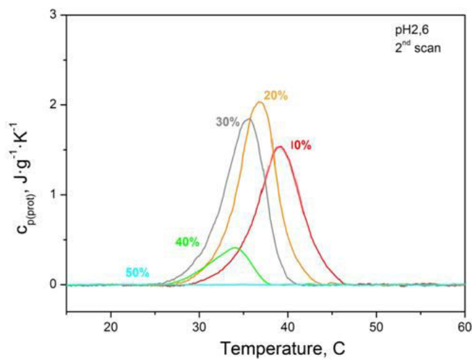
სურათი 3.3. გამეორებული სკანირების შედეგად მიღებული \alpha -ქიმოტრიპსინის თერმული ლლობის კალორიმეტრული მრუდები ხსნარში DMSO-ს სხვადასვა კონცენტრაციის პირობებში (ფოსფატის ბუფერი, pH 2.6, 0.05 NaCl).
