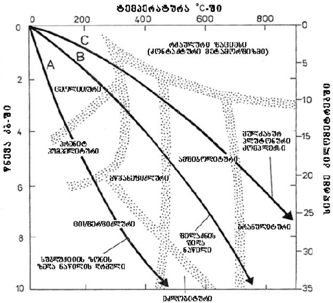
სურ. 5. მეტამორფული ფაციესები ვ. ერნსტის [61] მიხედვით. ისრებით ნაჩვენებია ტემპერატურის მატება სიღრმესთან ერთად, ჩ. პლამერისა და დ. მაკგერის [60] მიხედვით. A – სუბდუქციური ზონის ზედა ნაწილის დარი, B – ფილაქნის შიდა ნაწილი, C – ვულკანურ-პლუტონური კომპლექსი.
