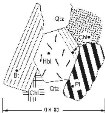
სურ.55. კვარც-დიორიტული ორთოგნეისის ჩანახატი მიკროზონდური კვლევისათვის (ნიმ.9, იხ. ცხრ.8)
